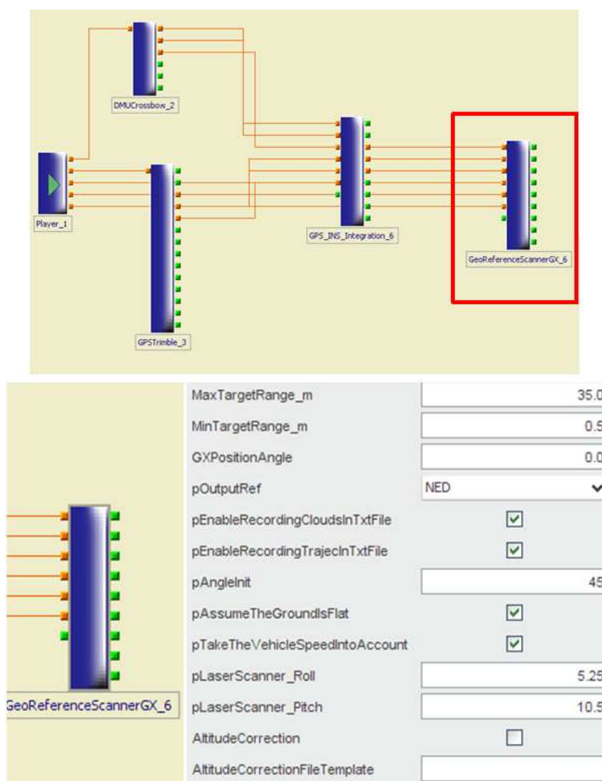
Figure 7-3 : Génération de nuage de points
