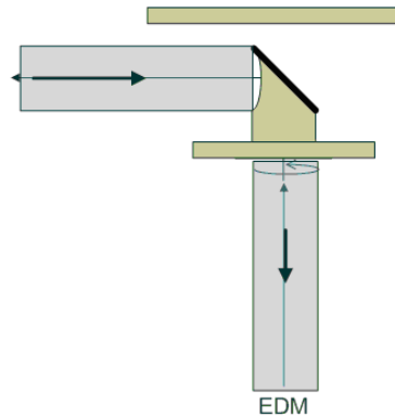
Figure 2-46 : Principe de déflexion du laser des scanners de LYNX et VQ-250
