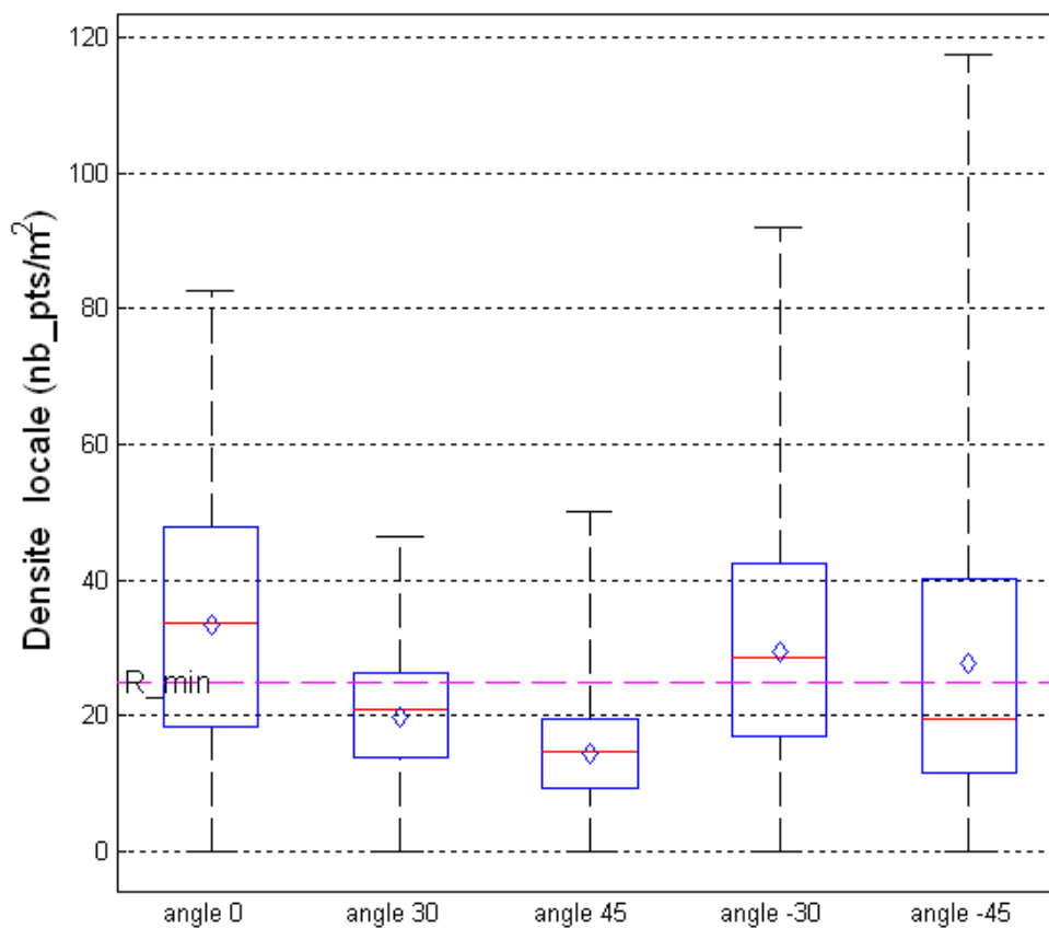
Figure 4-12 : Résolution de différents relevés selon l'angle de lacet
