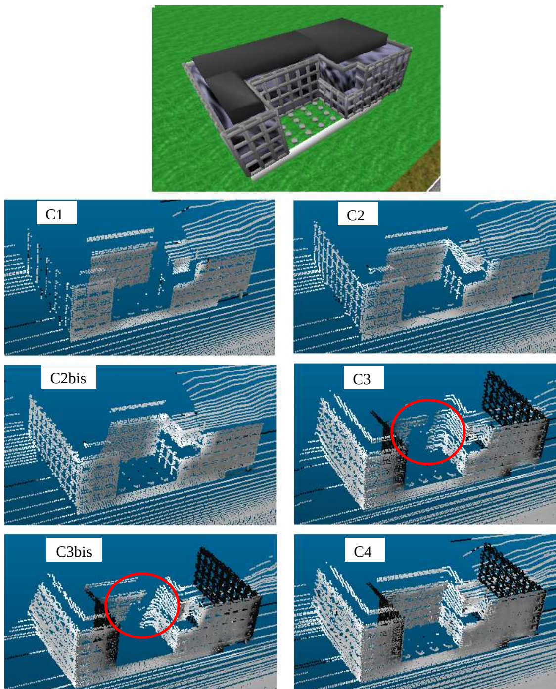
Figure 5-17 : Surface couverte sur un bâtiment en U
