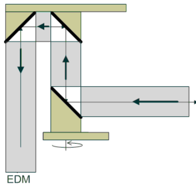
Figure 2-46 : Principe de déflexion du laser des scanners de LYNX et VQ-250
