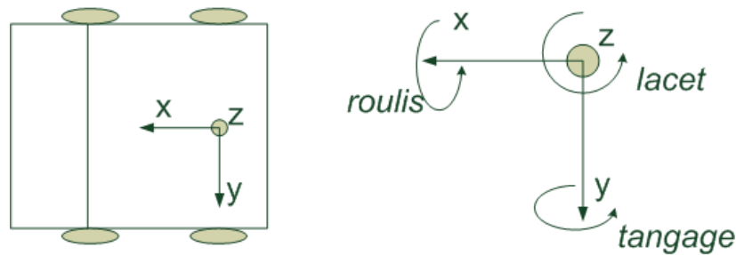
Figure 4-1 : Repère local de la plateforme
