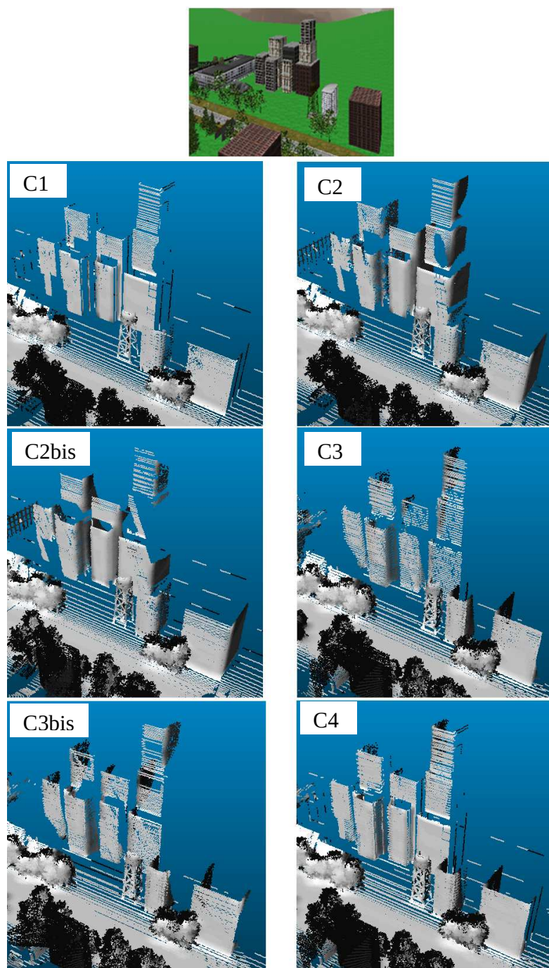
Figure 5-18 : Surface couverte sur un bâtiment lointain
