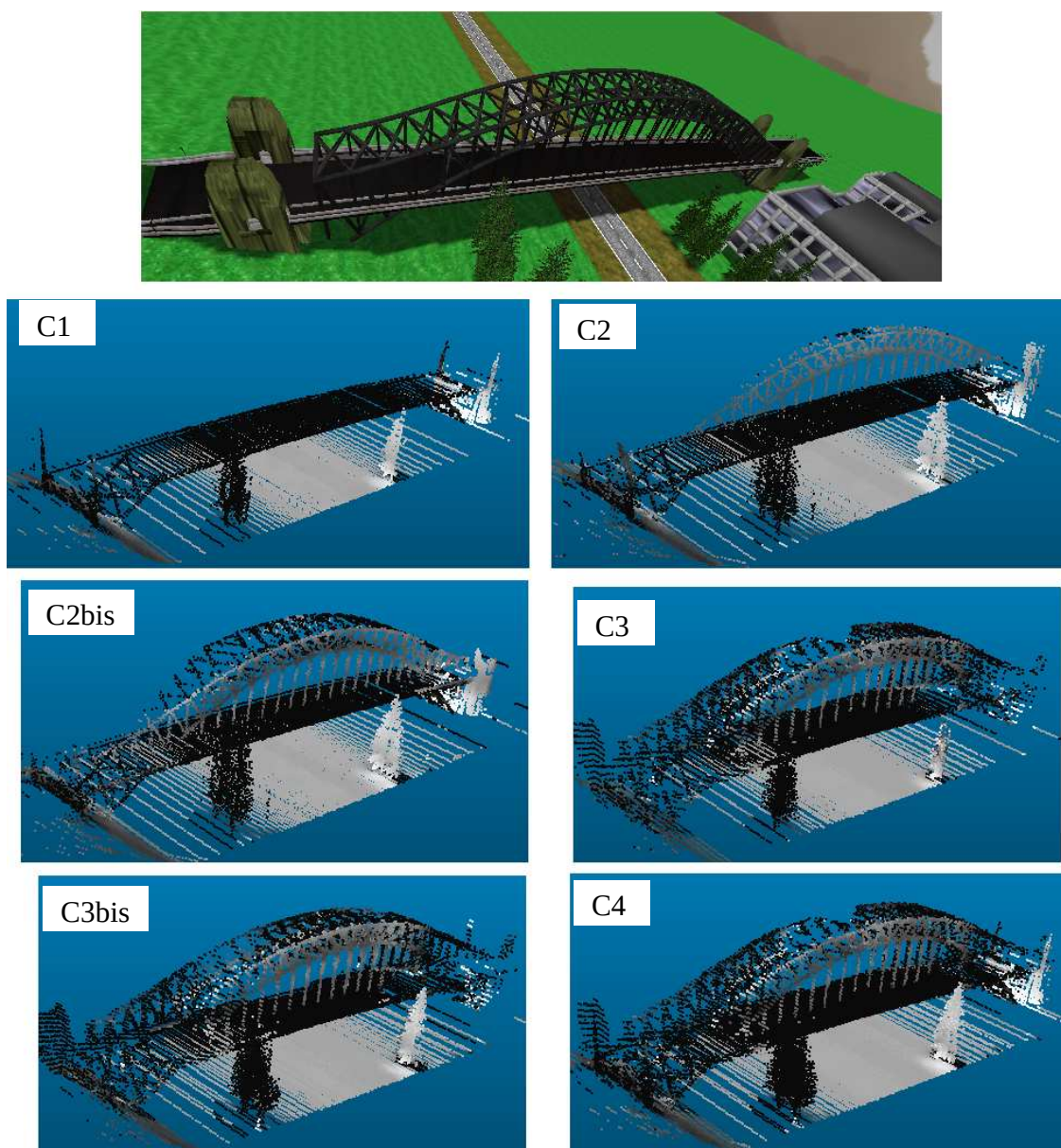
Figure 5-19 : Surface couverte sur un pont
