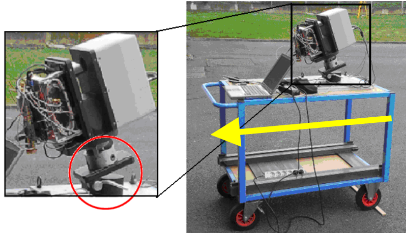
Figure 4-13 : Scanner mono-plan sur chariot
